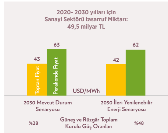
Geçmişte gözlemlenen elektrik fiyatları ve önümüzdeki dönemde farklı senaryolara göre fiyatların (USD/MWh) seyri ve muhtemel tasarruflar
