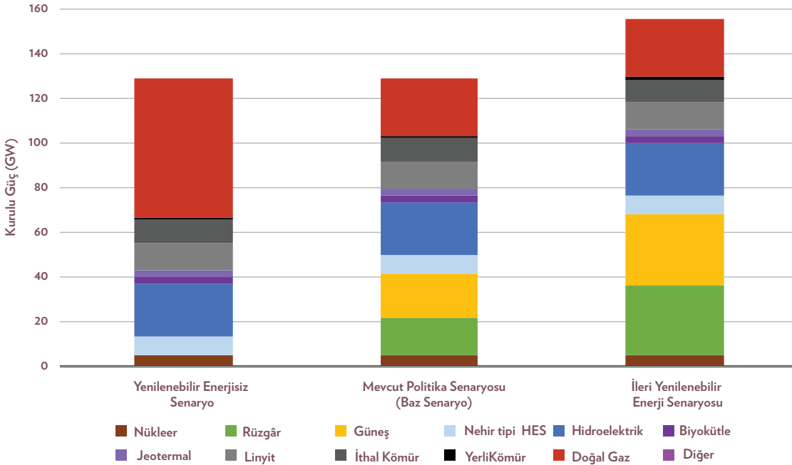
Farklı senaryolar altında 2030 yılı elektrik kurulu gücü (GW)
